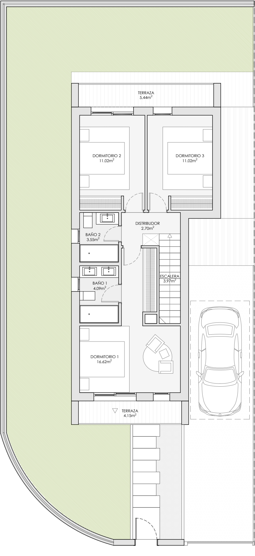
PLANTA PRIMERA
