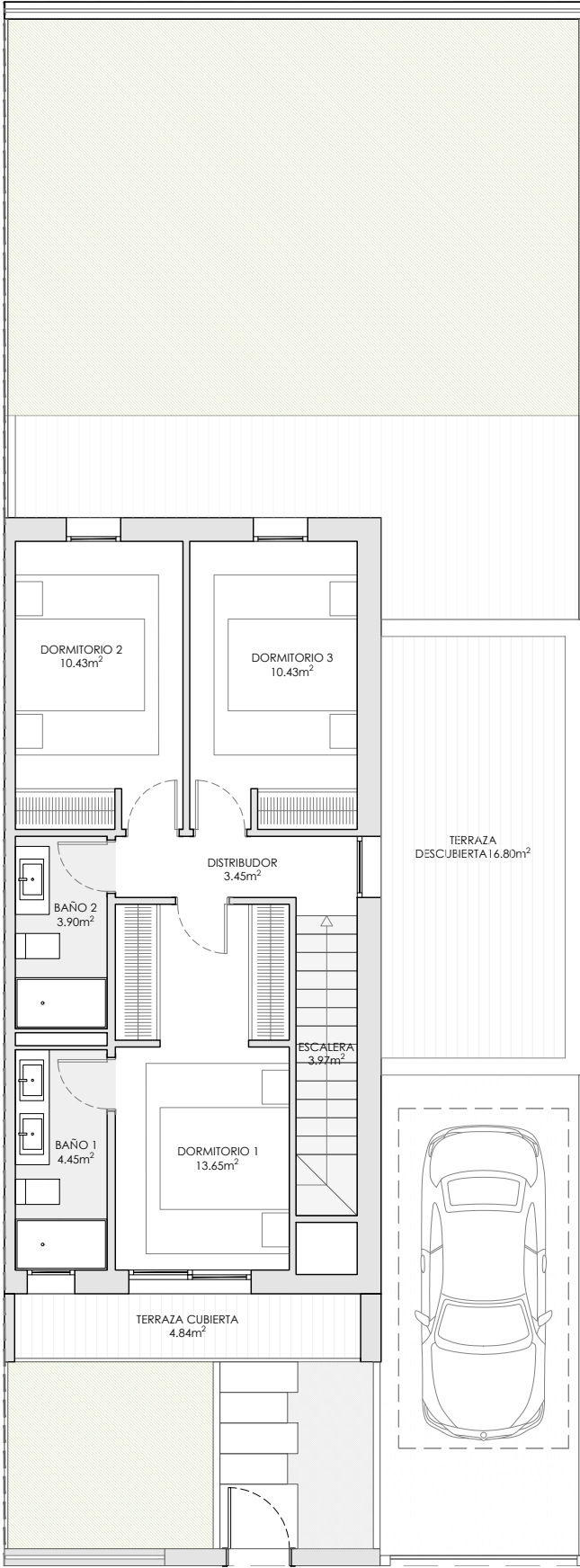
PLANTA PRIMERA
