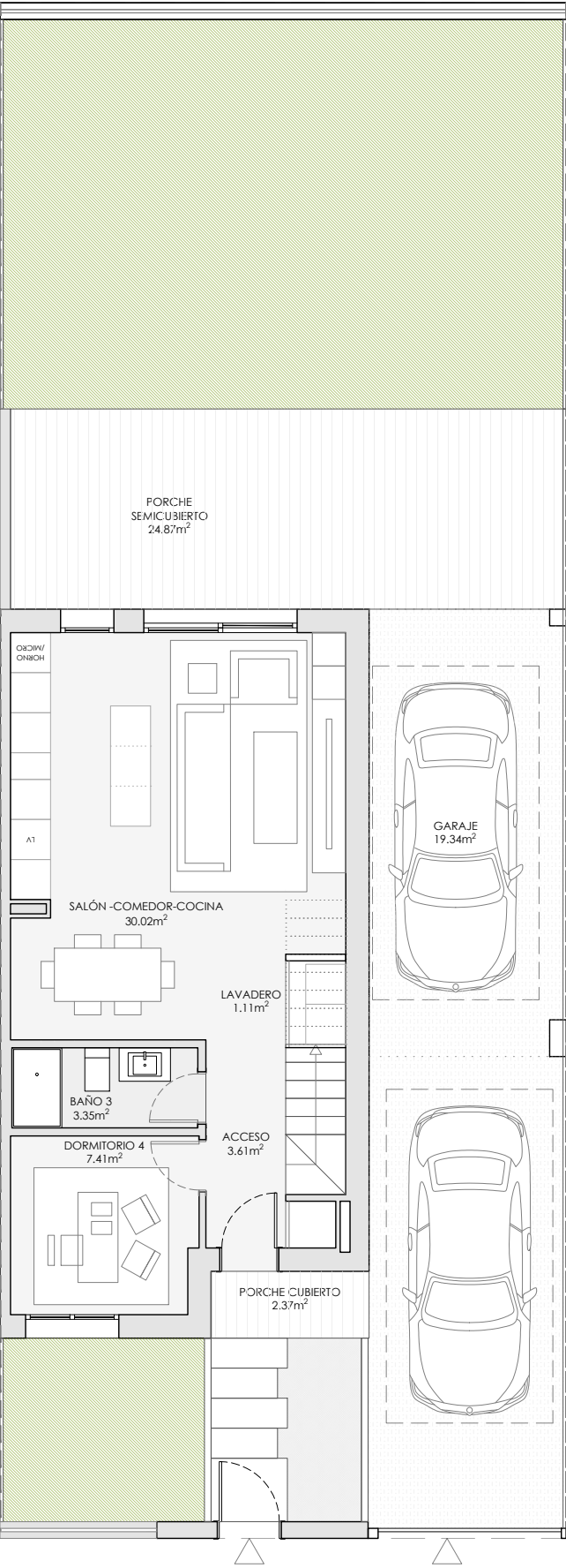
PLANTA BAJA
